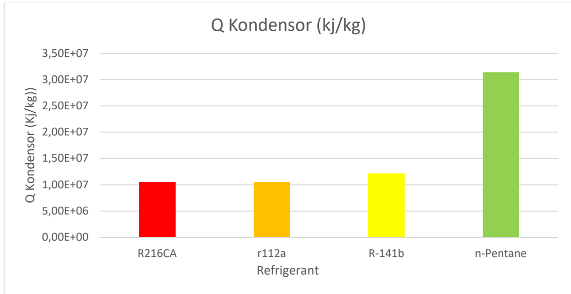
Gambar 5. Grafik Perbandingan Q Kondensor ORC
